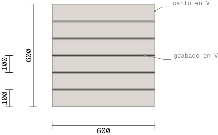
EN PLANTA, DESDE ABAJO · LA CARA DEL PLAFÓN
